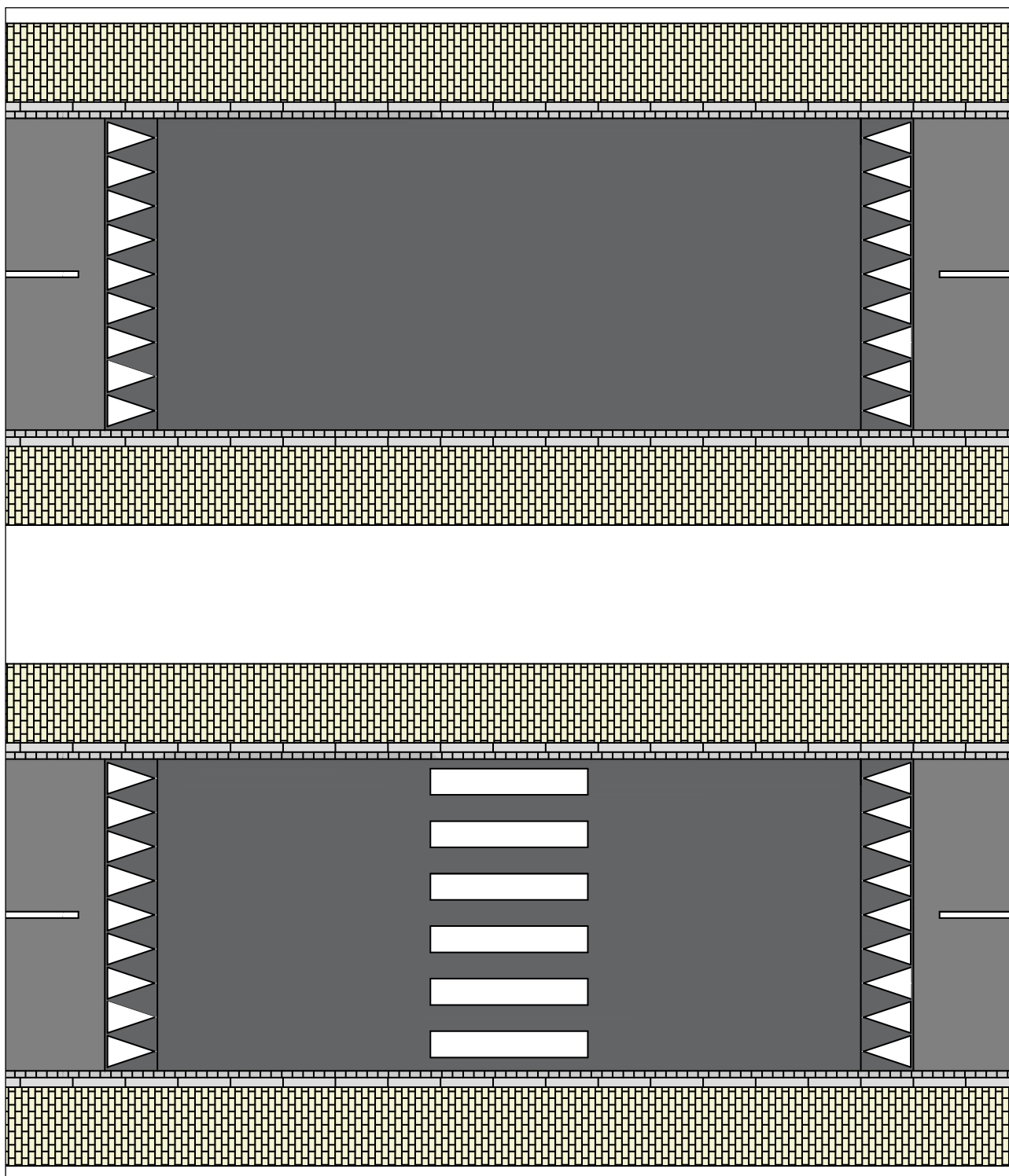
Ralentisseur type «plateau» (option : traversée pour piétons resp. cyclistes c.-à-d. gué ou passage)
