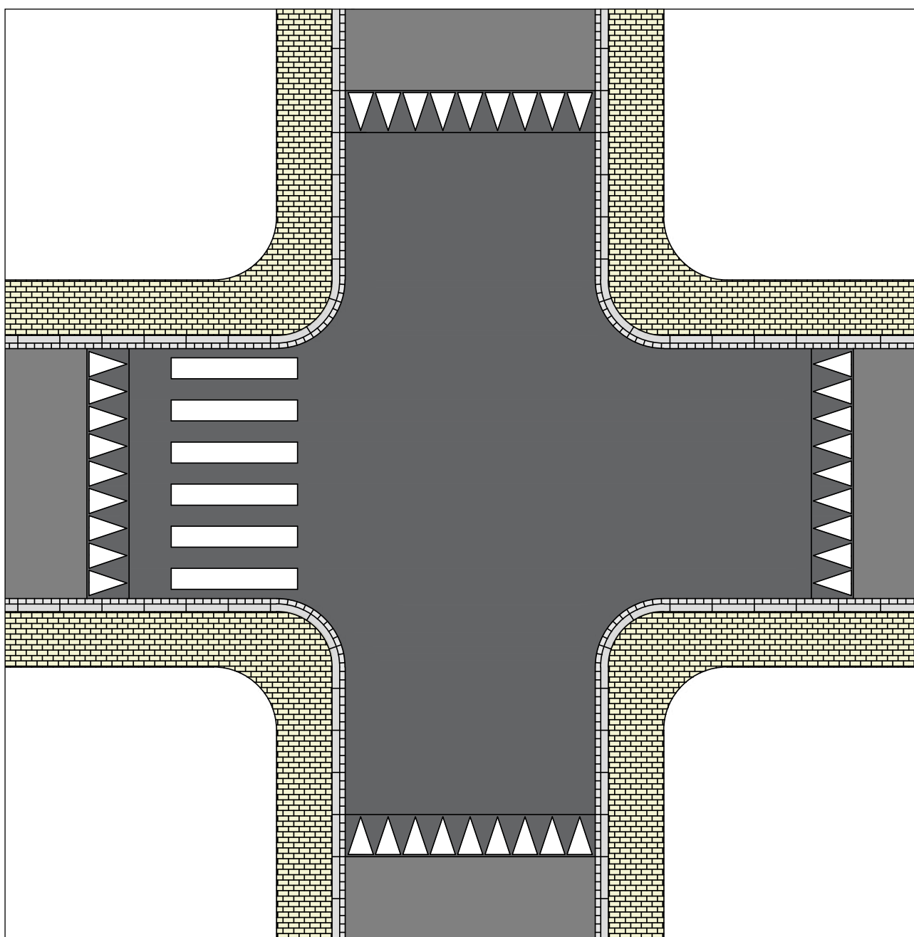
Ralentisseur type « carrefour surélevé » (option : traversée pour piétons resp. cyclistes c.-à-d. gué ou passage)
