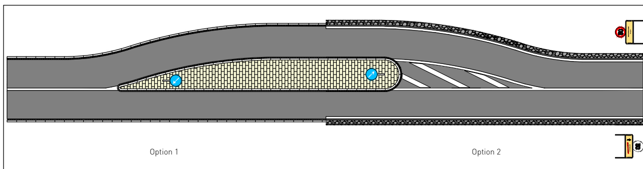
Chicane asymétrique à îlot ou terre-plein central
