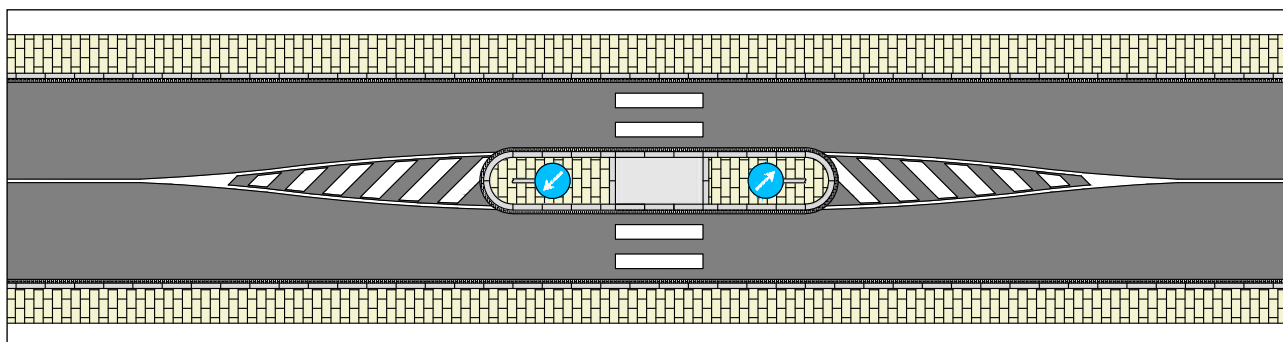
Îlot médian (option : traversée pour piétons resp. cyclistes c.-à-d. gué ou passage)
