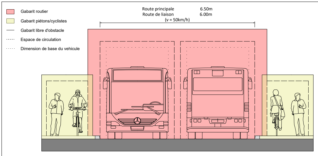
Chaussée réduite aux dimension minimales (cas avec 50 km/h)
