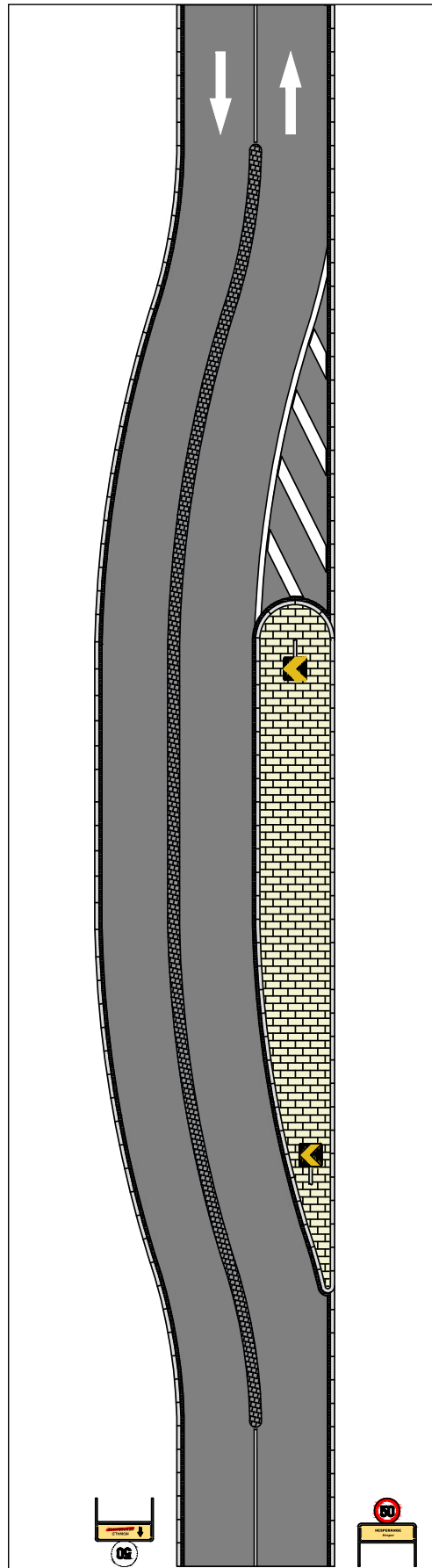
Chicane latérale à îlot
