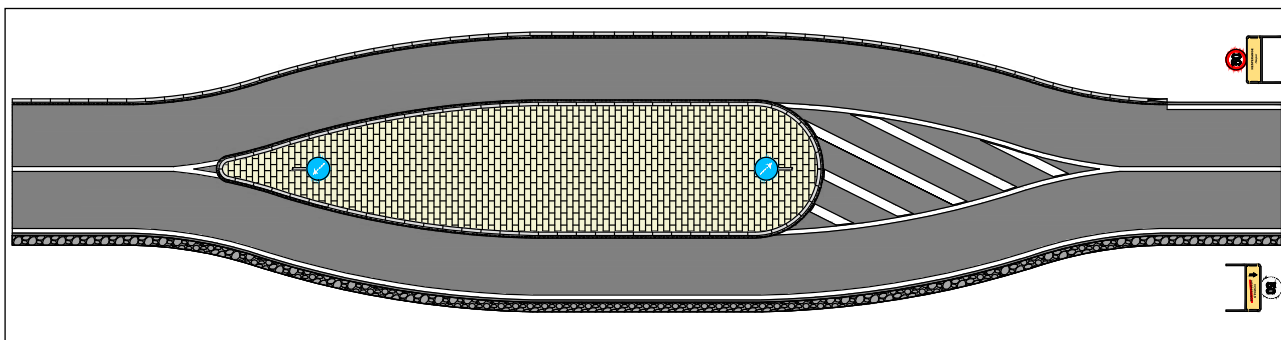
Chicane symétrique à îlot ou terre-plein central
