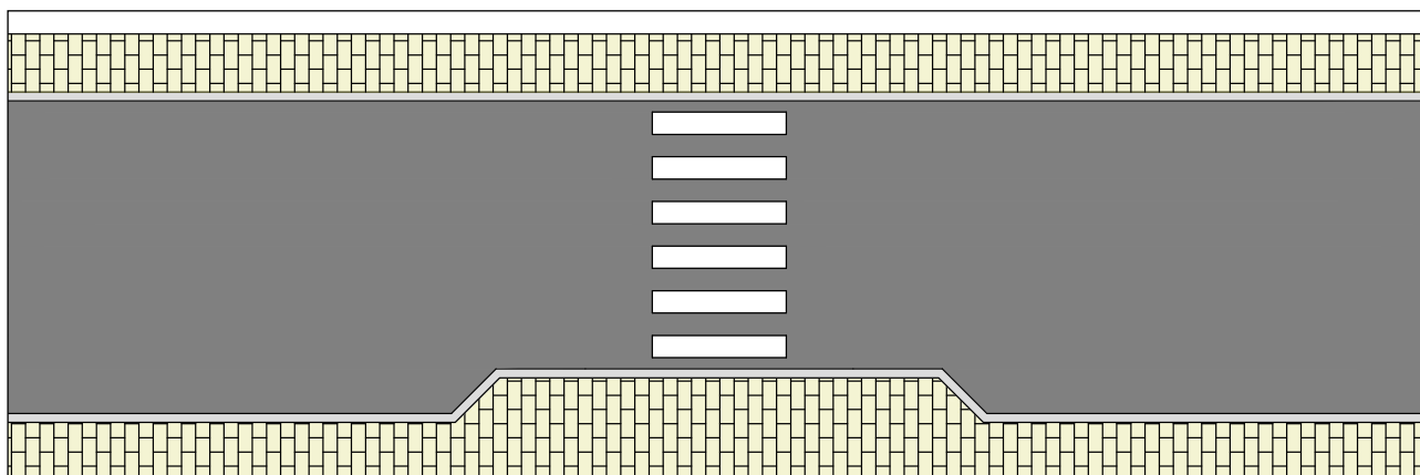
Rétrécissement latéral de la chaussée – avec traversée pour piétons
