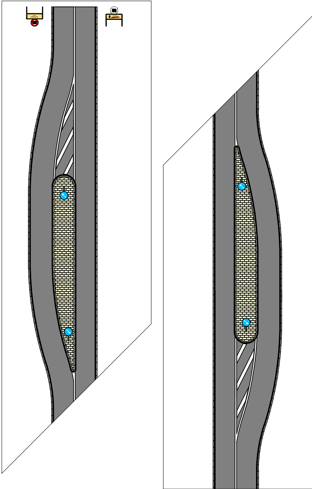
Chicane asymétrique à îlot ou terre-plein central
