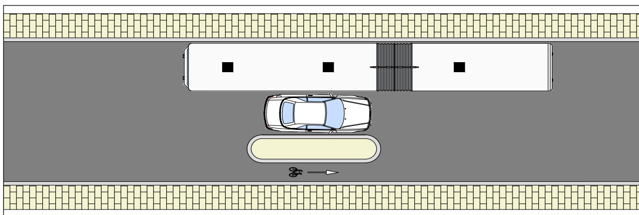
Rétrécissement latéral de la chaussée – avec bypass pour cyclistes
