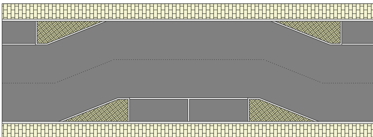
Décrochement horizontal – avec emplacements de stationnement
